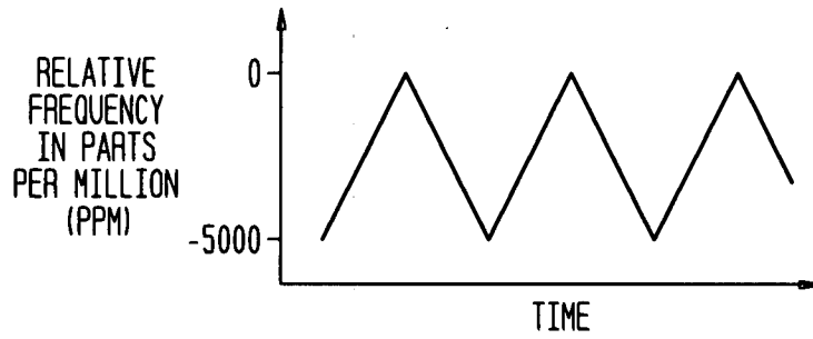
FIG. 2A TX
