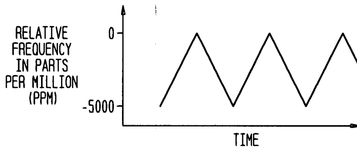
FIG. 2B RX
