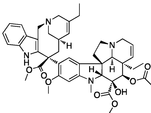
Vinorelbine
