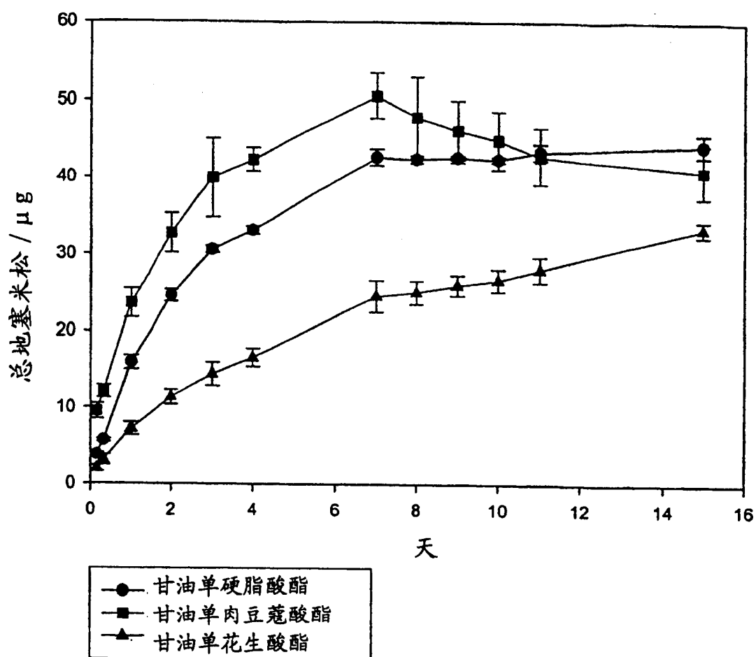
图 2: 单酸甘油酯中地塞米松的释放 (n=3)
