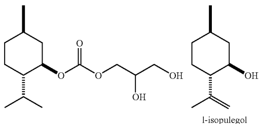
l-isopulegol
