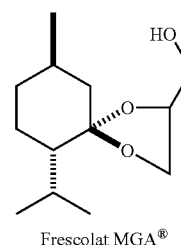
Frescolat MGA ®
