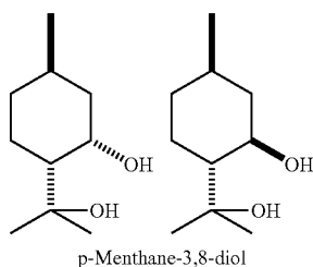
p-Menthane-3,8-diol
