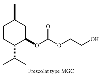
Frescolat type MGC
