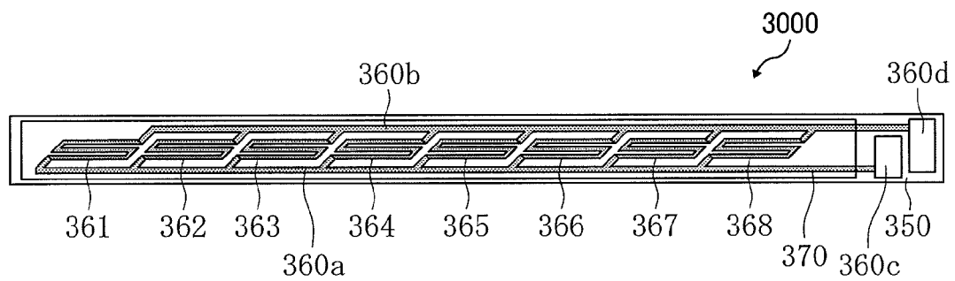
FIG. 3L
