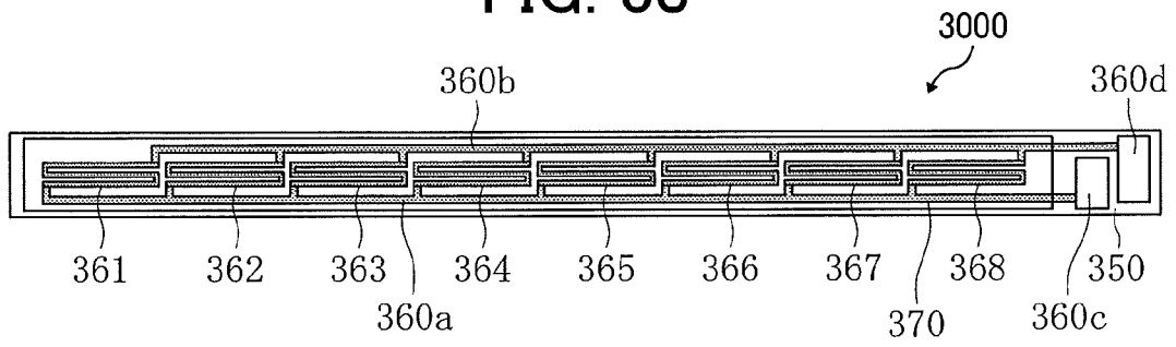
FIG. 3J
