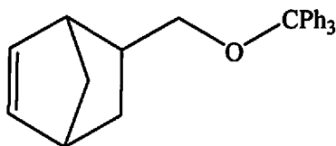
10 NBMeOCPh 3
