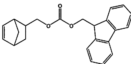
NBMeOFMOC
