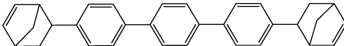
5 10 15 20 25 30 4,4''-di(bicyclo[2.2.1]hept-5-en-2-yl)-1,1':4',1''-terphenyl.
