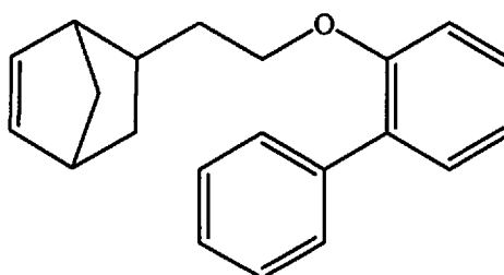
NBEtO-2-PhPh
