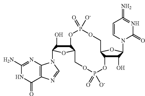
c-GpCp
