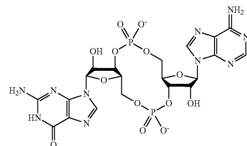
c-GpAp
