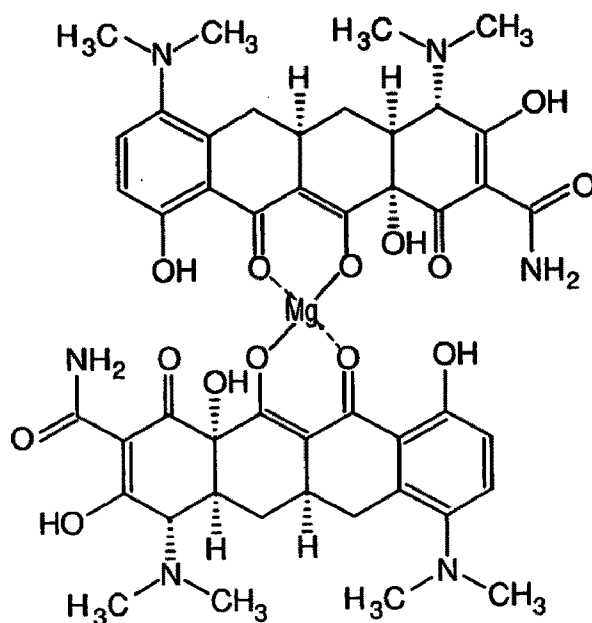
Bis(minocyclinato)magnesium
