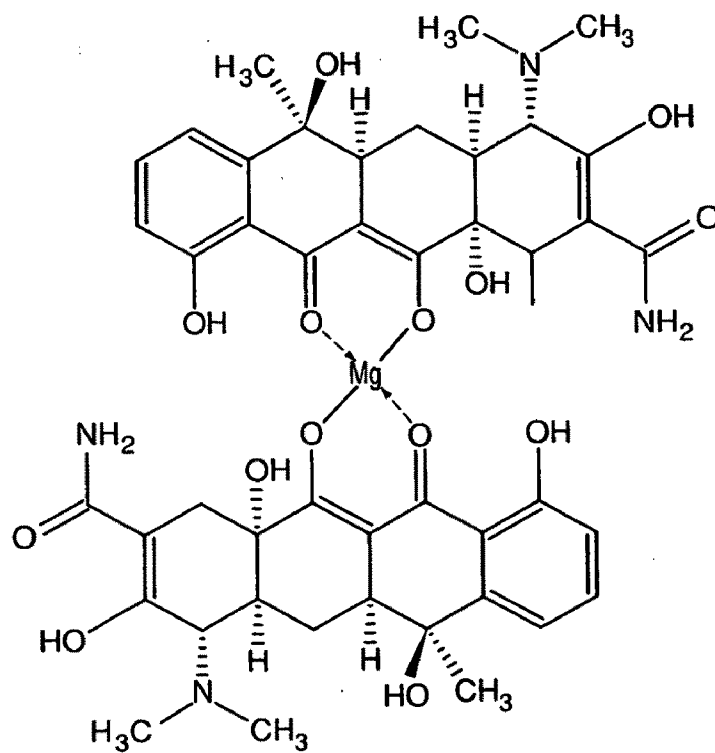
Bis(tetracyclinato)magnesium
