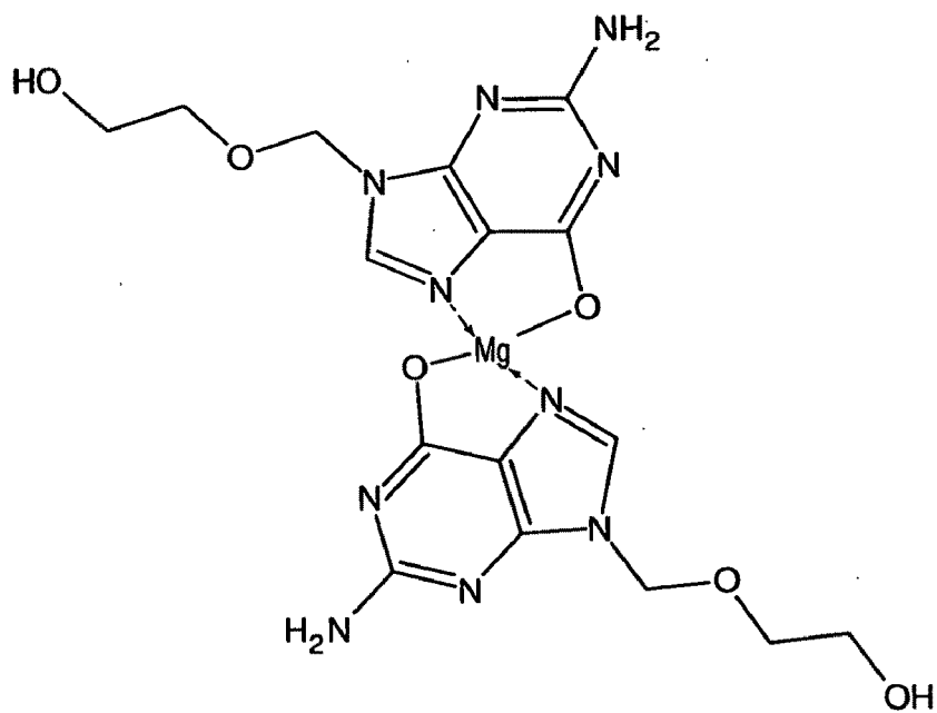
Bis(acycloguanosinato)magnesium
