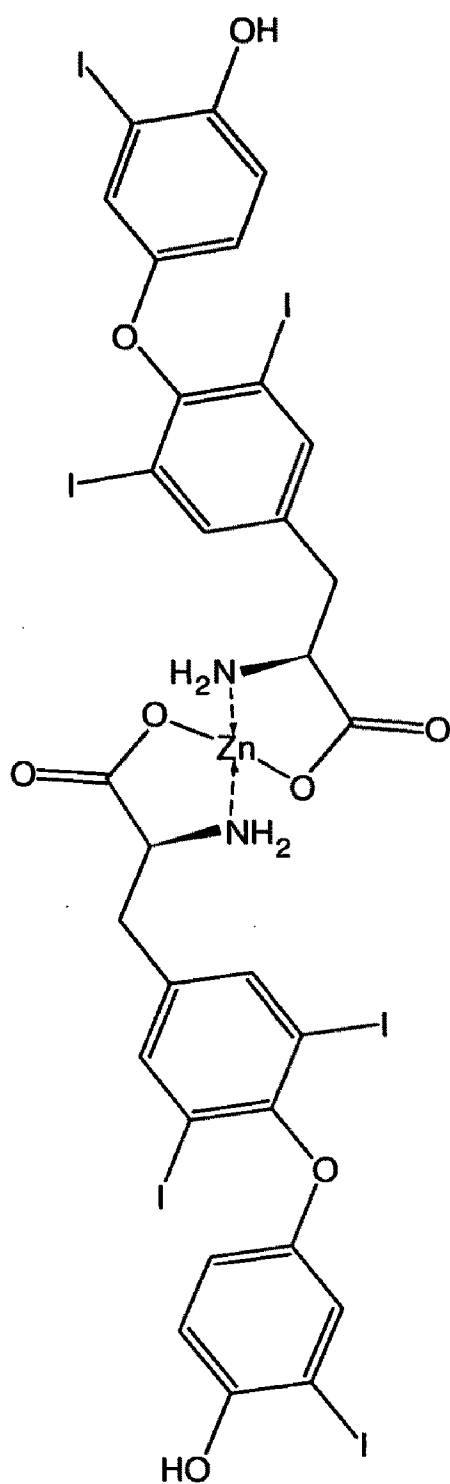
Bis(triiodothyroninato)zinc
