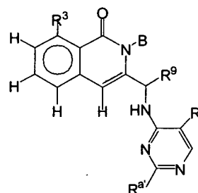
Formula XIV-A
