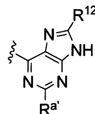
Formula III(d)
