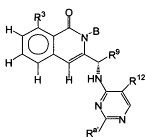
Formula XIV-A2
