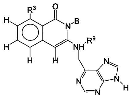
Formula VI-A
