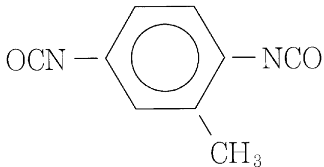
toluene 2,5 - diisocyanate (Desmodur T)
