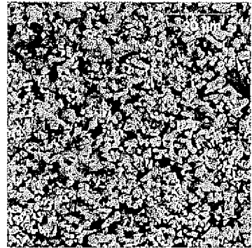
FIG. 20C 0.5 Hrs @1600°C
