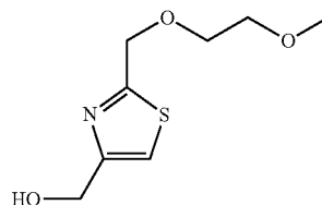
(2-((2-Methoxyethoxy)methyl)thiazol-4-yl)methanol
