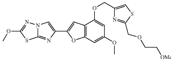
Example 6. 2-Methoxy-6-(6-methoxy-4-((2-((2-methoxyethoxy)methyl)thiazol-4-yl)methoxy)benzofuran-2-yl)imidazo[2,1-b][1,3,4]thiadiazole
