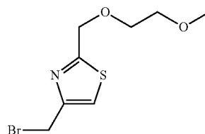
6E. 4-(Bromomethyl)-2-((2-methoxyethoxy)methyl)thiazole
