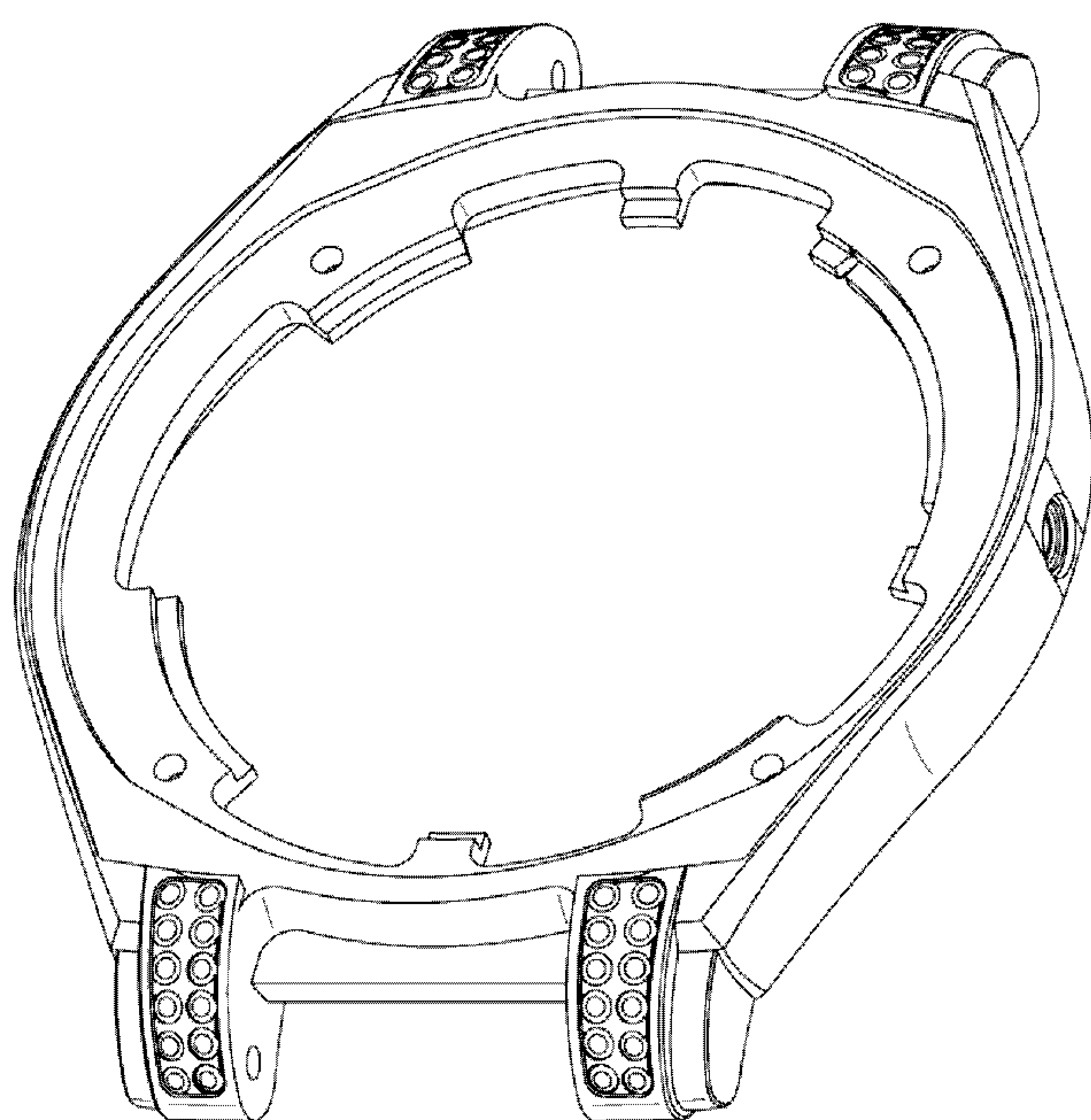
【立體圖】
