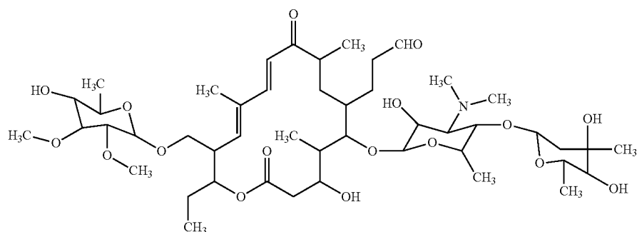
Tylosin A.
