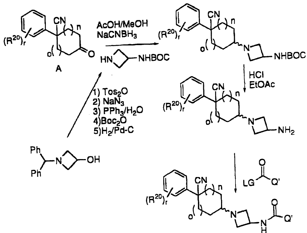
Scheme 1 (cont'd)
