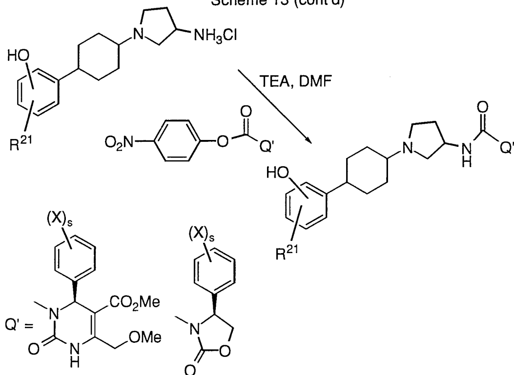
Scheme 13 (cont'd)
