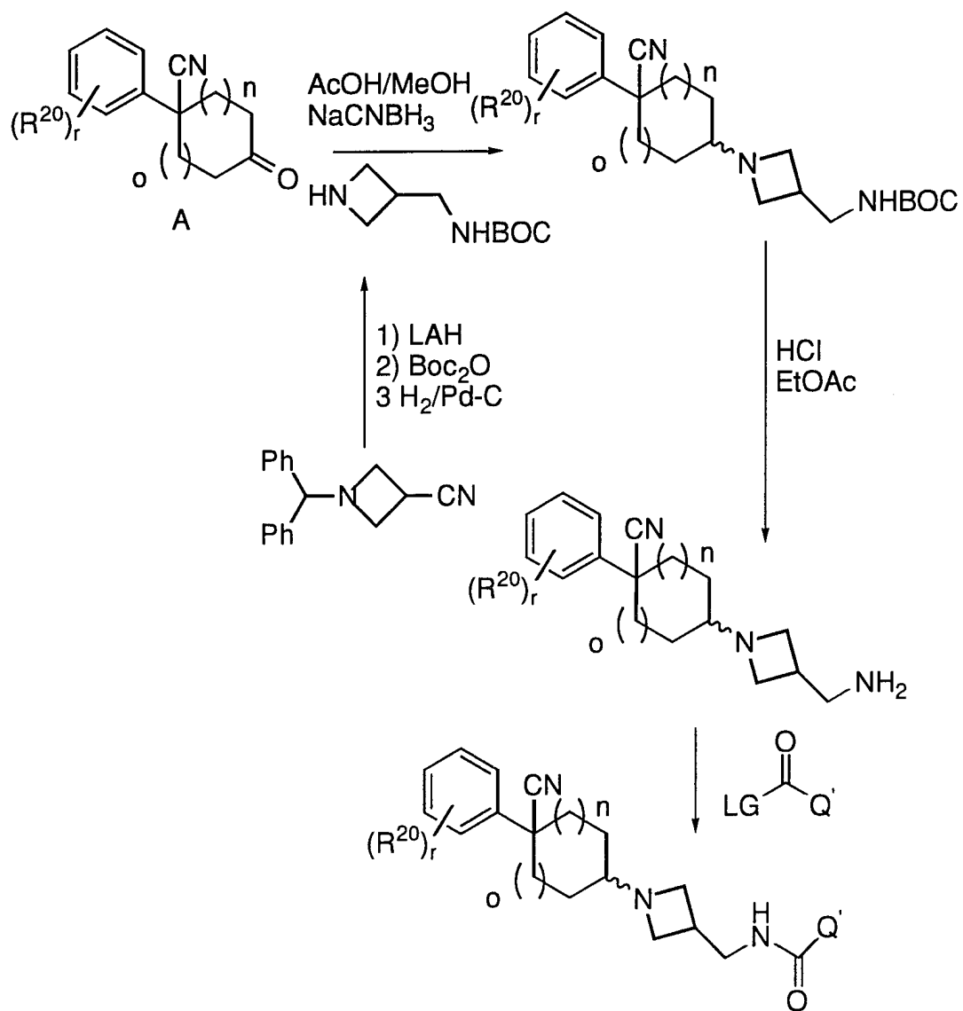
Scheme 1 (cont'd)
