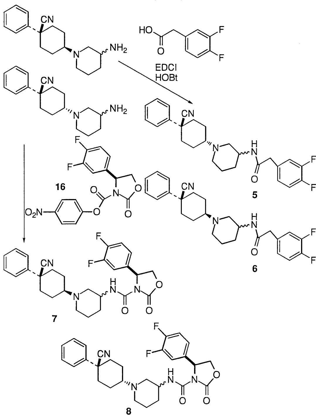
Scheme 3 (cont'd)
