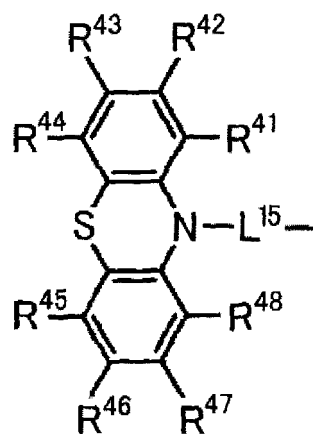
allgemeine Formel (6)
