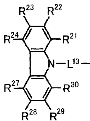
allgemeine Formel (4)
