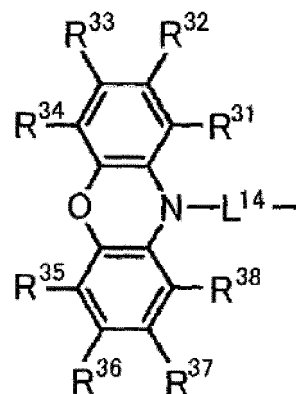
Formule générale (5)
