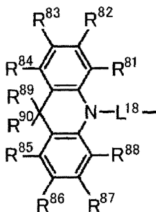
Formule générale (8)
