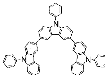
Tris-PCz
