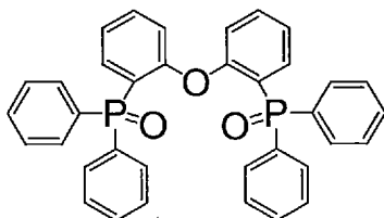
DPEPO
