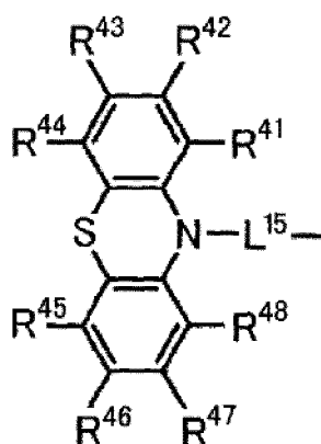
Formule générale (6)
