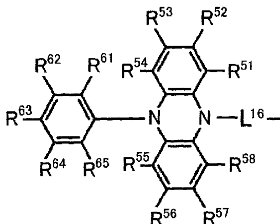
allgemeine Formel (8),
