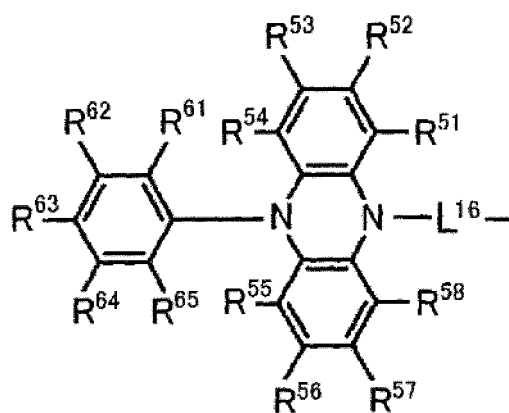
Formule générale (8)
