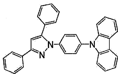
PzCz
