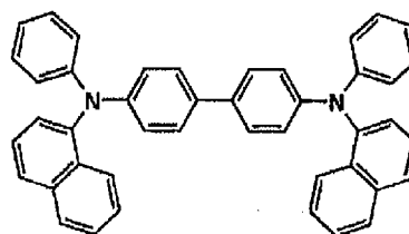
\alpha -NPD
