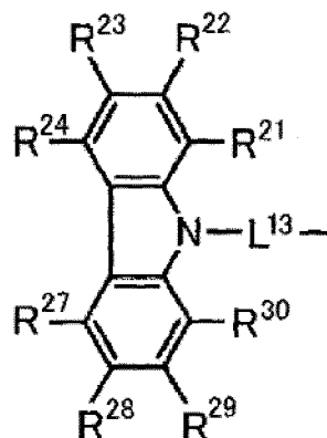
Formule générale (4)
