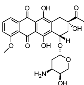
daunorubicin
