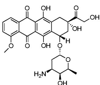
doxorubicin
