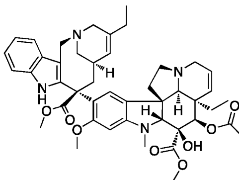
Vinorelbine
