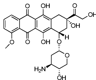
epirubicin
