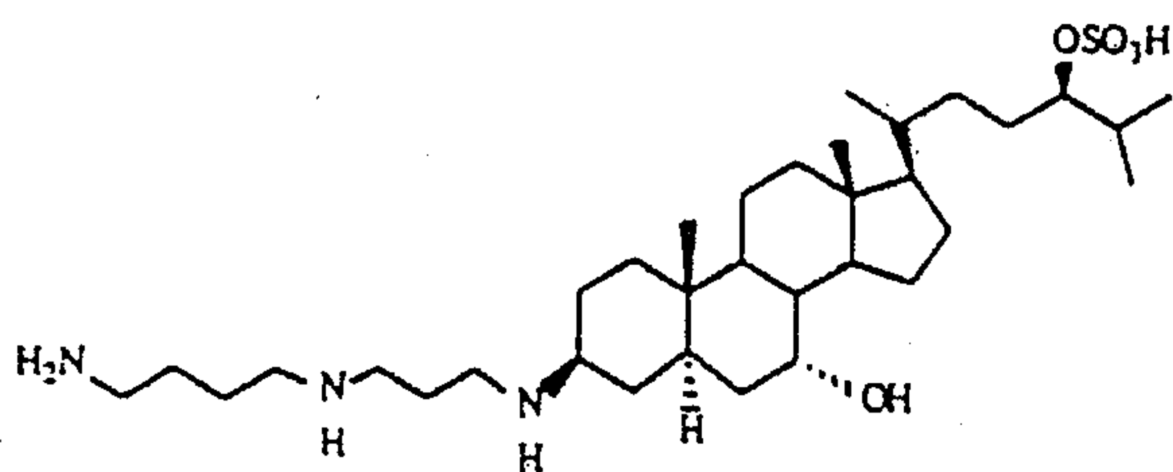
MSI- 1256
