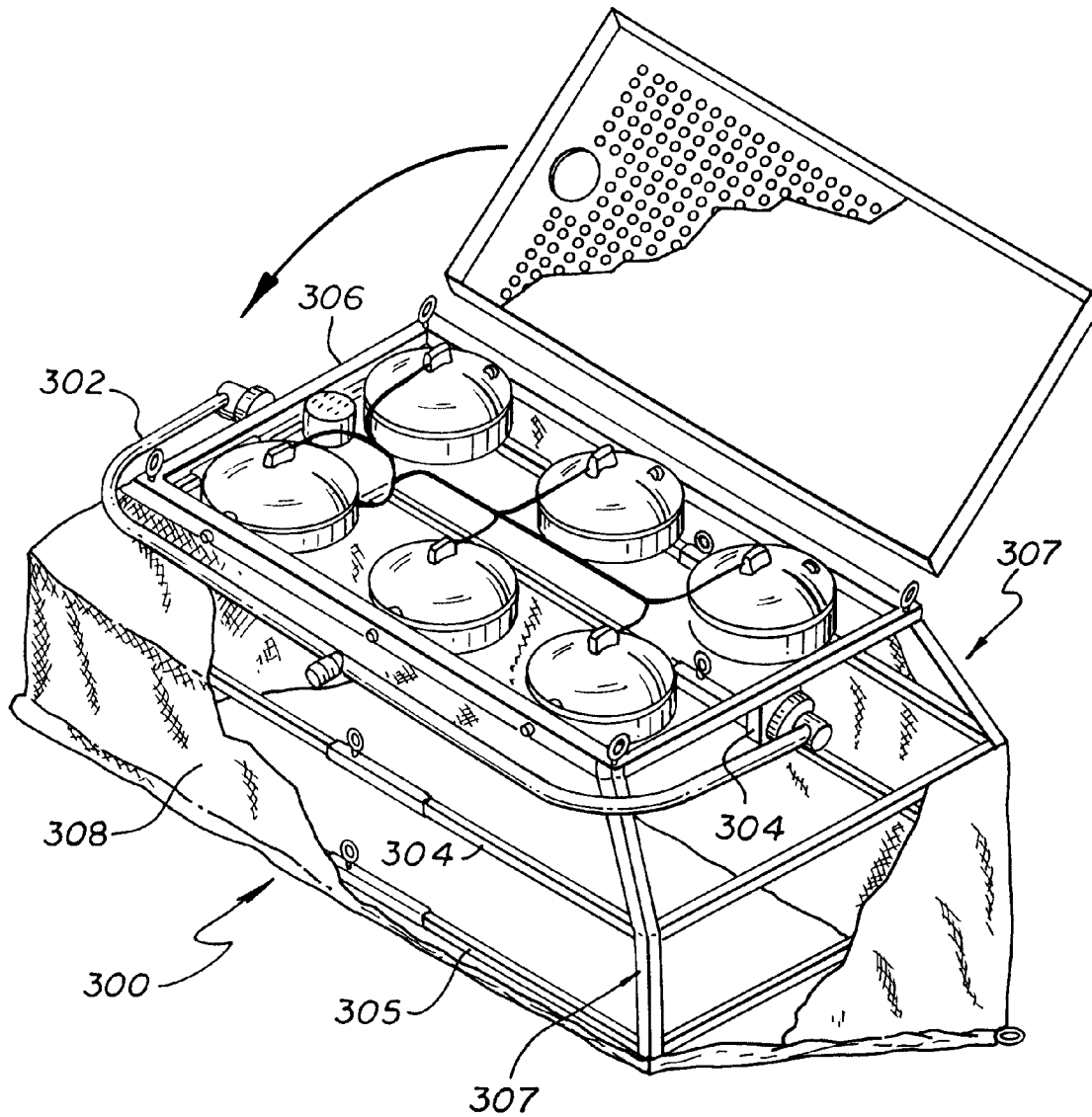
FIG. 42
