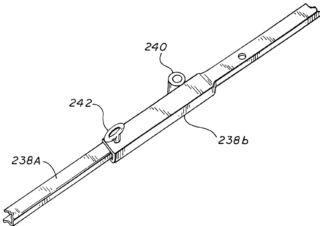
FIG. 34A
