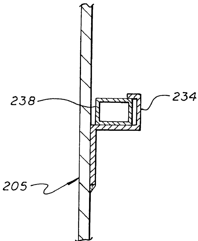
FIG. 37
