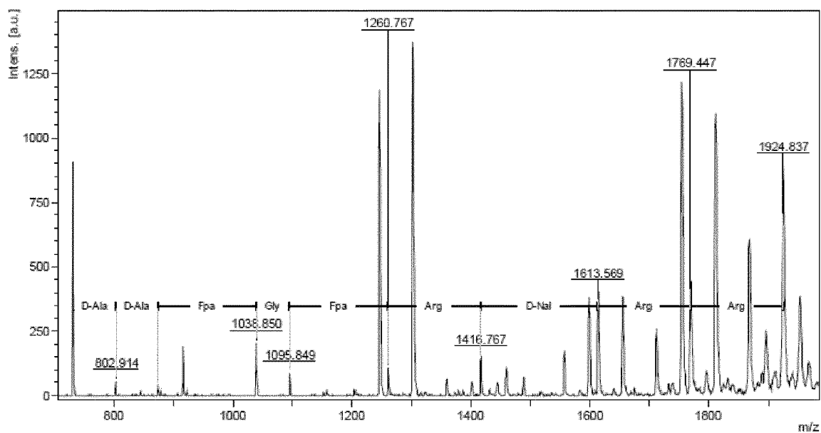
Cyclorasin 4A: cyclo(Arg-Arg-nal-Arg-Fpa-Gly-Fpa-ala-ala-Gln)
