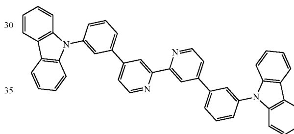
4,4'mCzP2BPy
