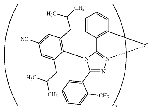
Ir(mpptz-diBiCNp) 3
