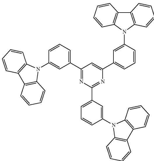
mCzP3Pm
