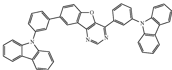
4,8mCzP2Bfpm
