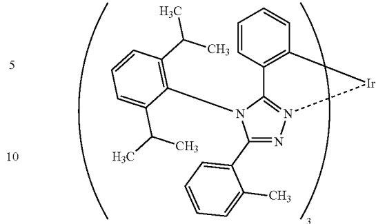
Ir(mpptz-diPrp) 3
