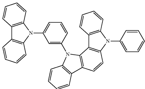
mCzPICz
