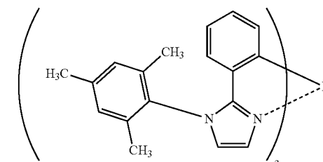
Ir(tmppim) 3
