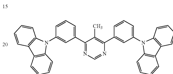
5Me-4,6mCzP2Pm
