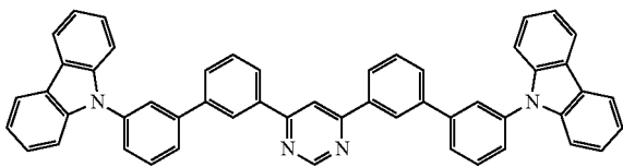
4,6mCzBP2Pm
