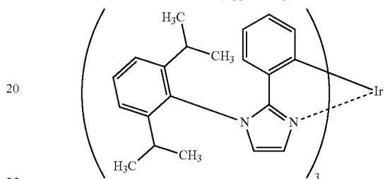
Ir(iPrpim) 3
