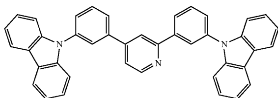
2,4mCzP2Py
