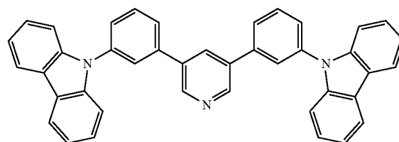
35DCzP2Py
