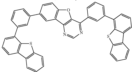
4,8mDBtP2Bfpm
