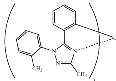
Ir(Mptz1-mp) 3
