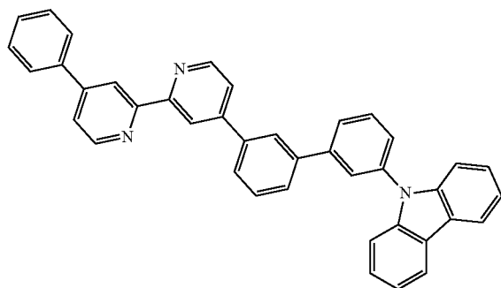
4'Ph-4mCzBPBPpy
