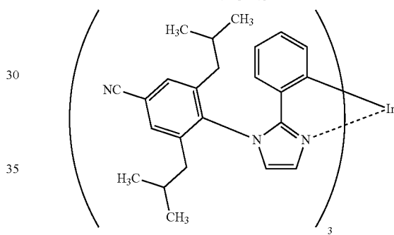
Ir(pim-diBiCNp) 3
