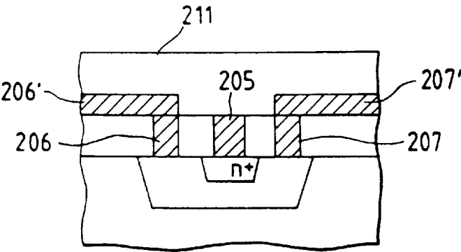
FIG. 10C
