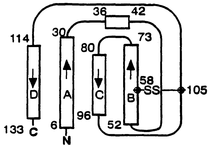
FIG. 2F IL-2
