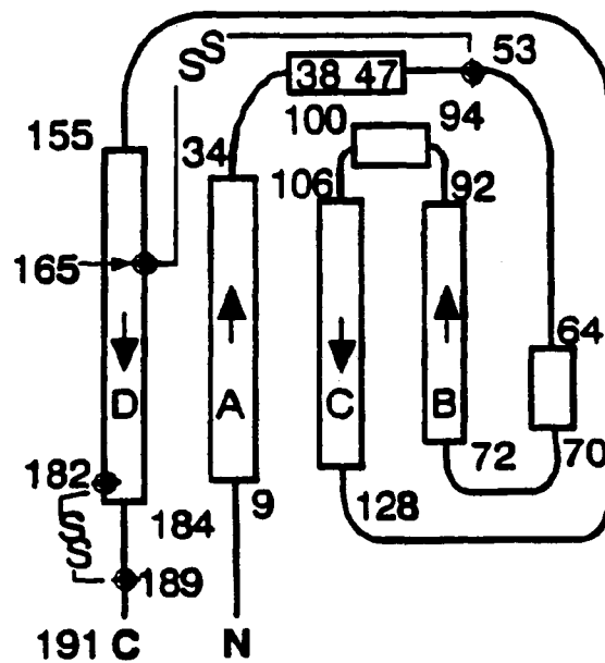
FIG. 2B hGH
