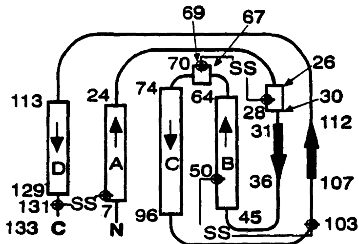
FIG. 2G IL-4
