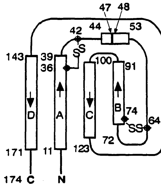
FIG. 2A rhG-CSF
