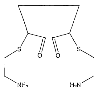
IXb
