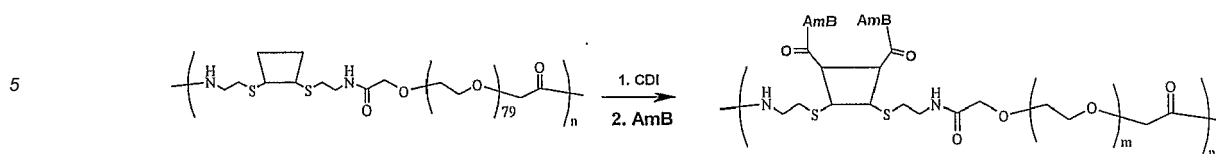
Scheme LII
