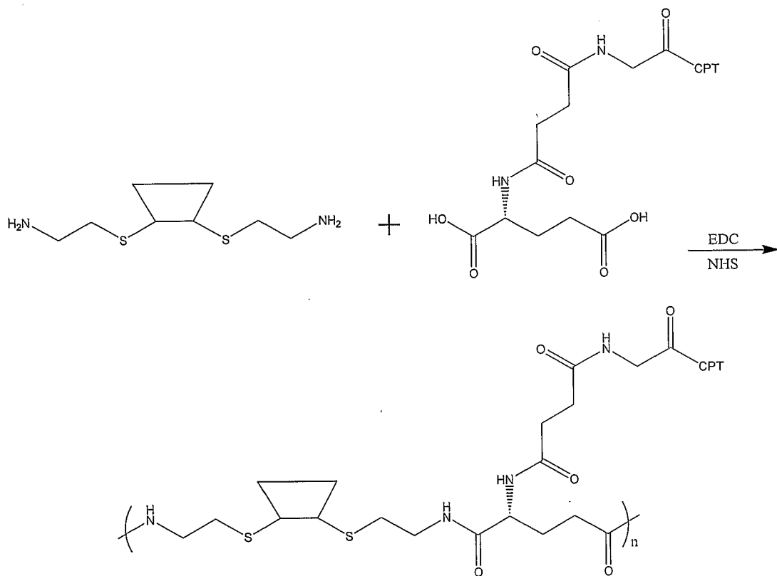
Scheme VI
