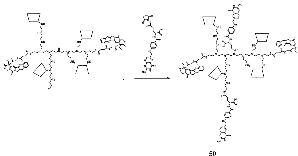
Scheme LI
