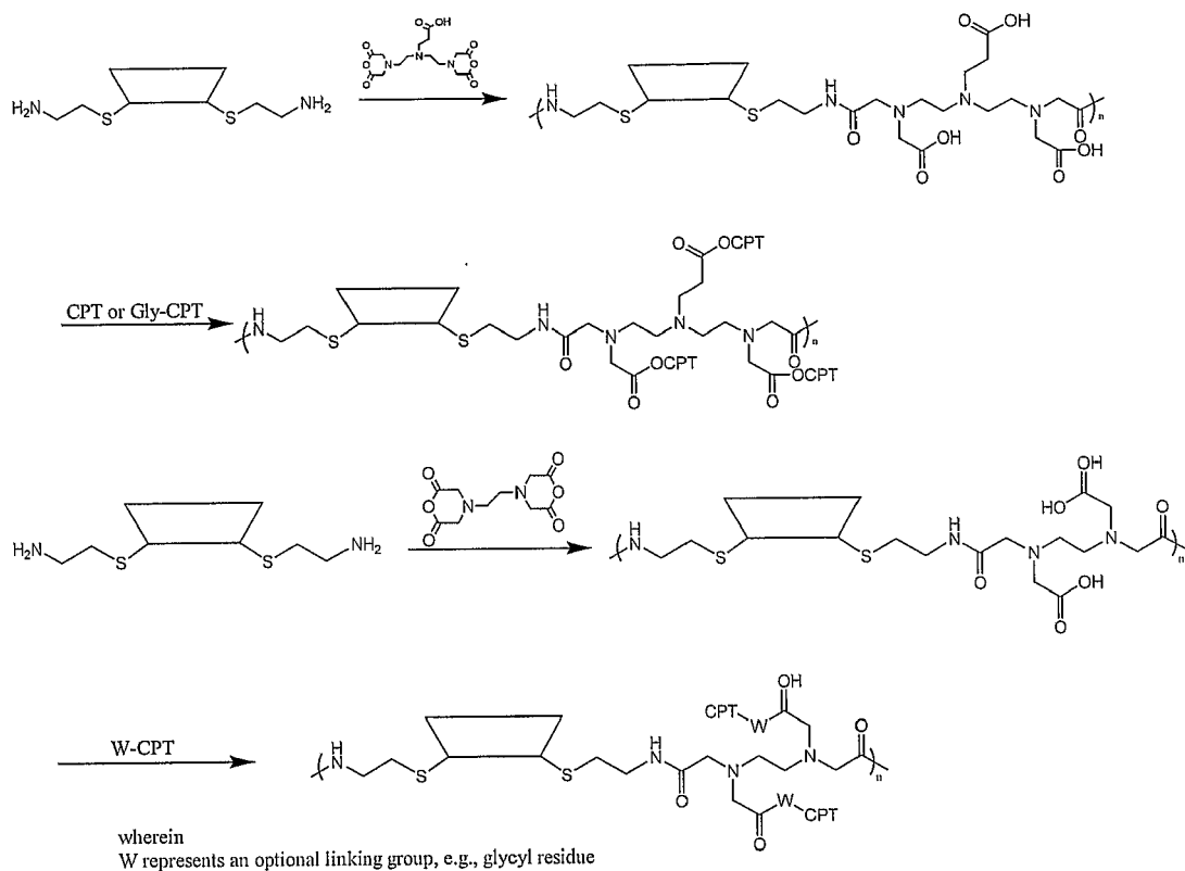
Scheme VI
