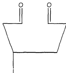
VIIc
