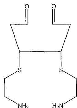
IXa
