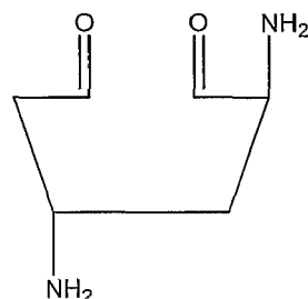
VIIIc
