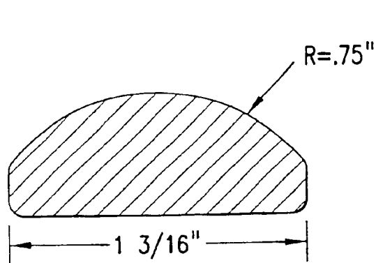
CATHODE FIG. 7A
