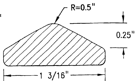
ANODE FIG. 7B
