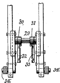
Fig. 7. on line 6-6.
