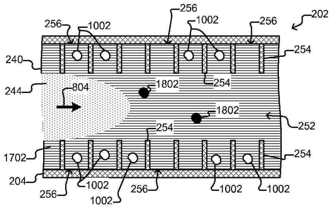
도면28
