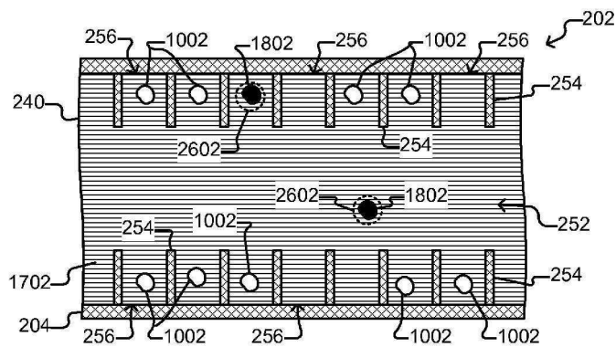
도면26
