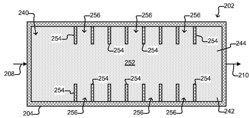
도면3a
