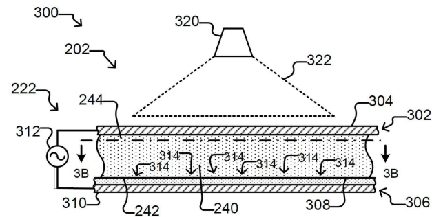
도면3a
