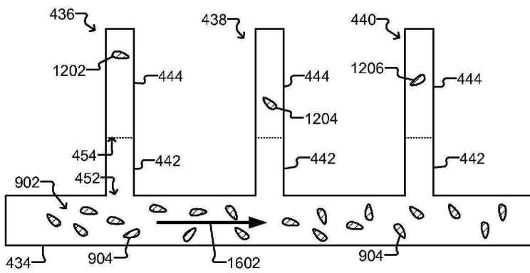
도면17
