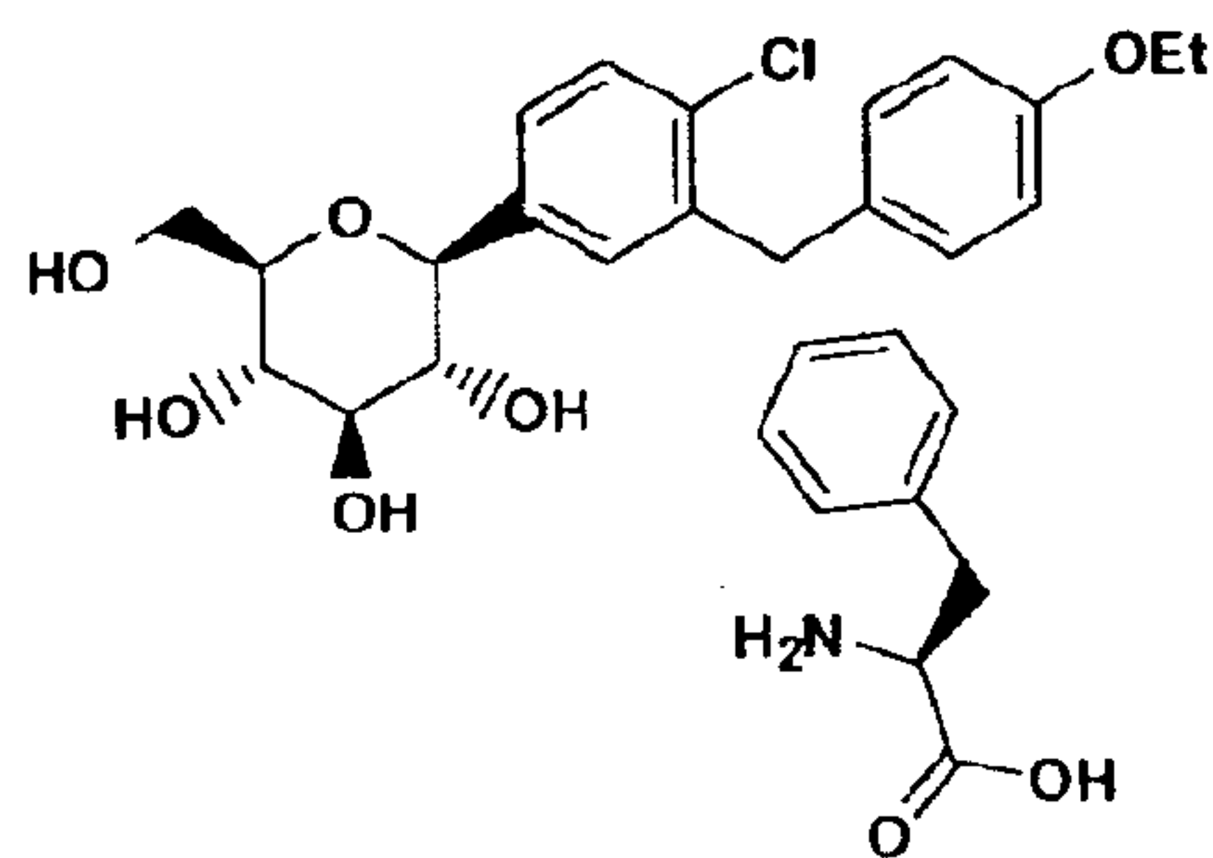
Compound Ik ; and
