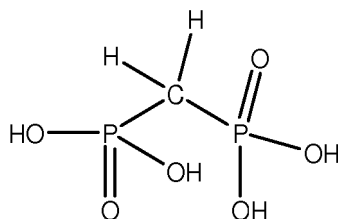
MDP
