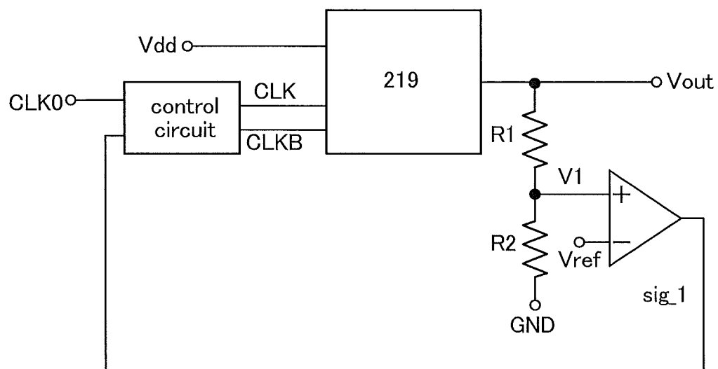
FIG. 22B
