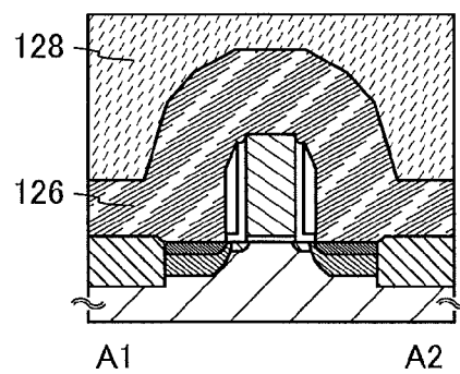
FIG. 3G
