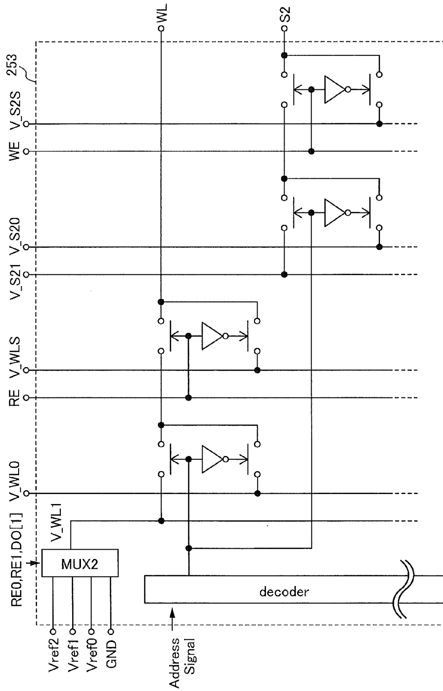
FIG. 29
