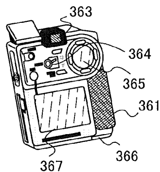
FIG. 32F
