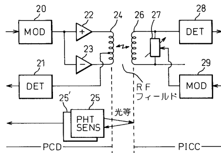
PICCとPCD間の通信インターフェースの一例
