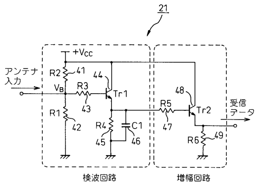
図 4 カード検波回路部の一実施例
