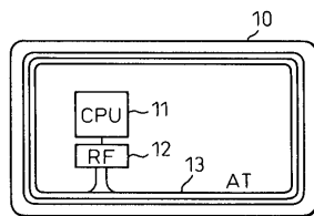
図 1 PICCの構成概要例
