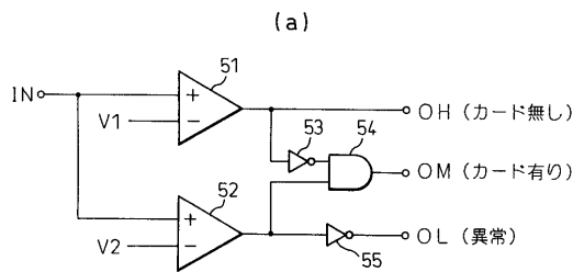
図 6 電圧検出回路部の一実施例
