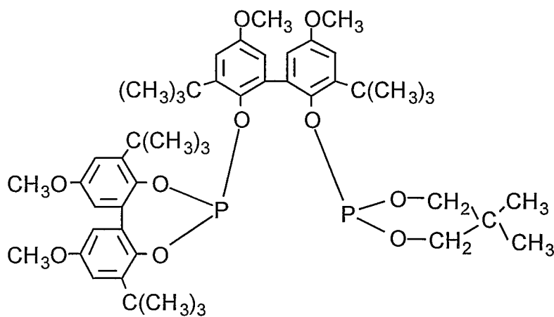
Ligand N
