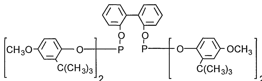
Ligand T
