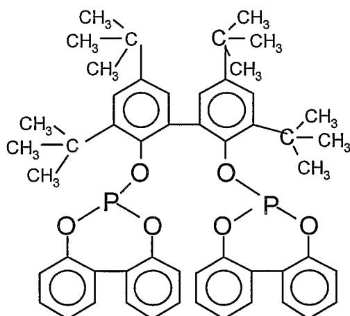
Ligand D
