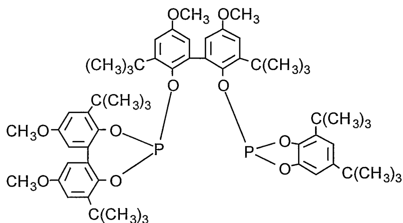
Ligand L
