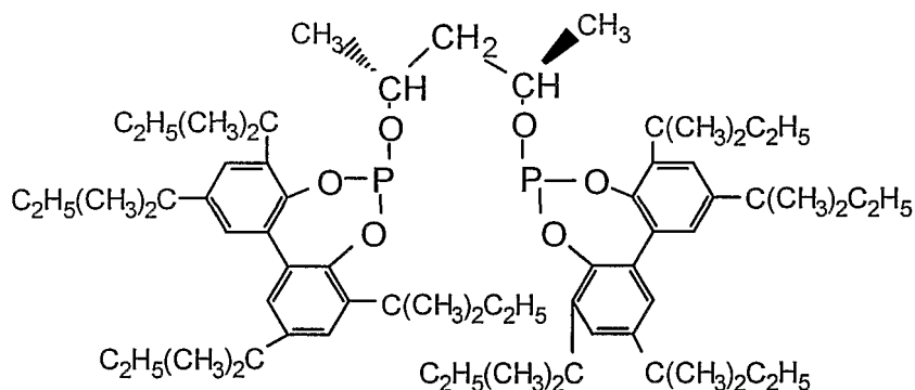
Ligand E
