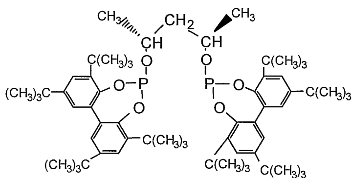
Ligand F
