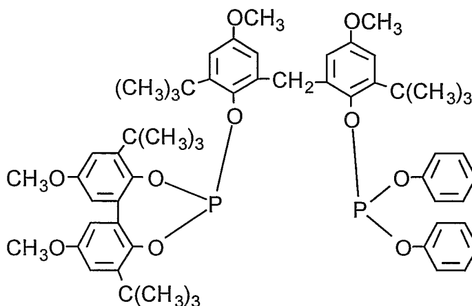
Ligand P
