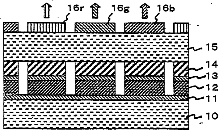
FIG. 3 Color Filter/Fluorescence Conversion Layer
