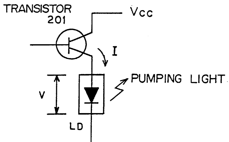
FIG. 23B
