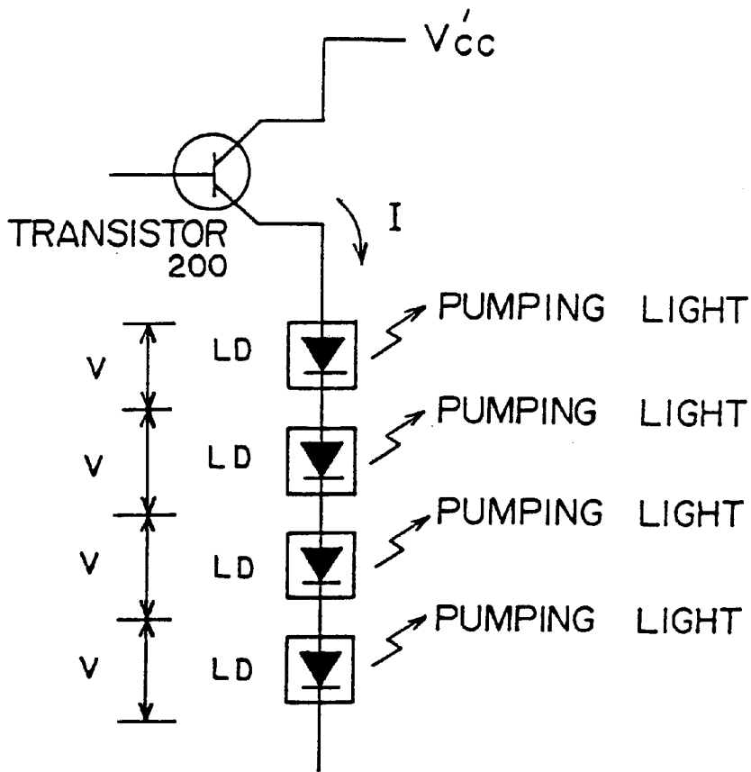
FIG. 23A
