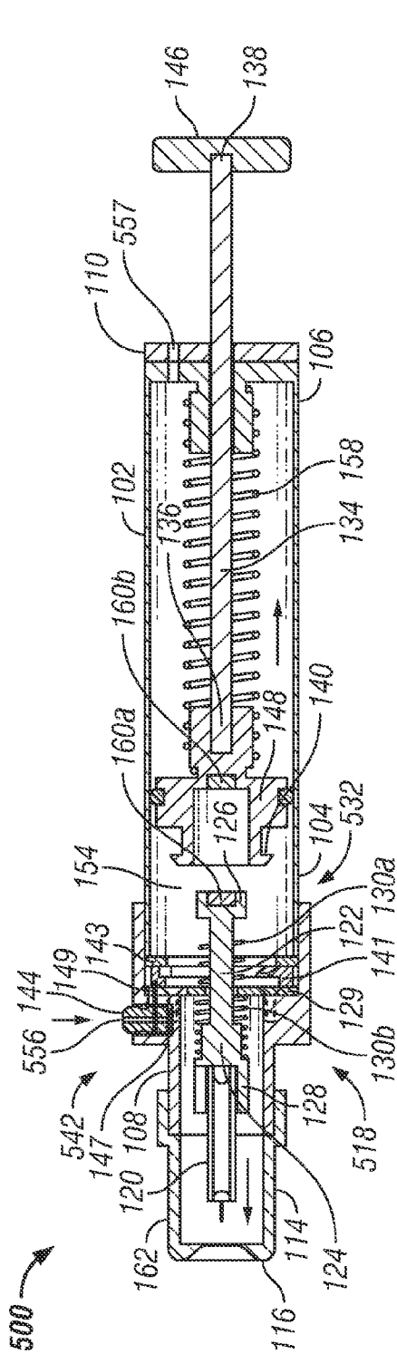
FIG. 15C
