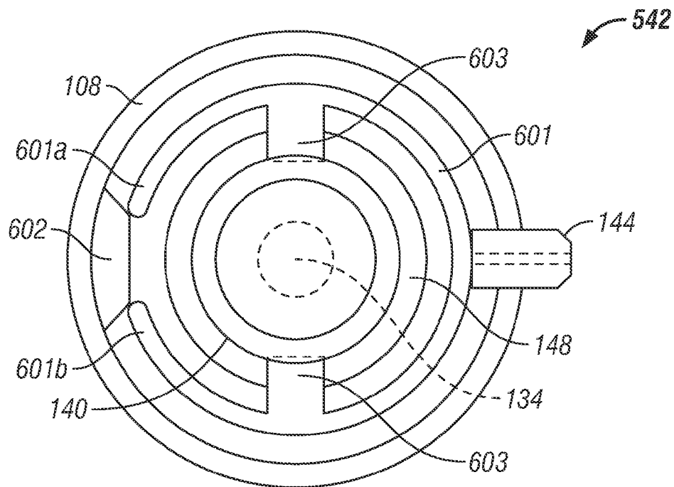
FIG. 14E
