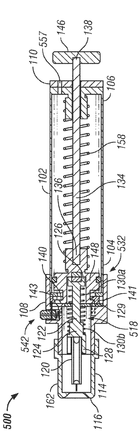
FIG. 15A
