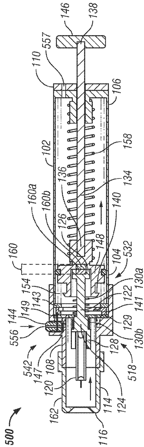
FIG. 15B
