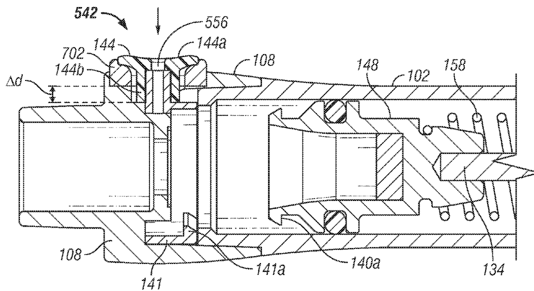
FIG. 14D
