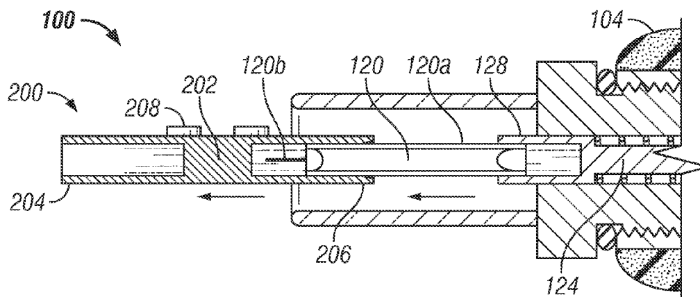
FIG. 8D
