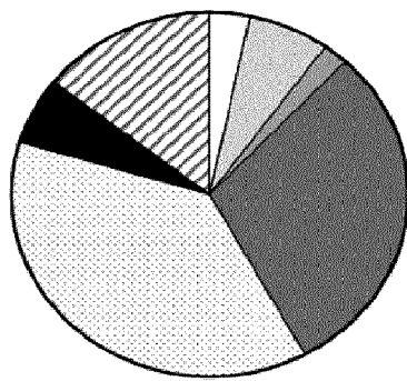
H5-VLP
