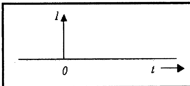
: Dirac Delta Function
