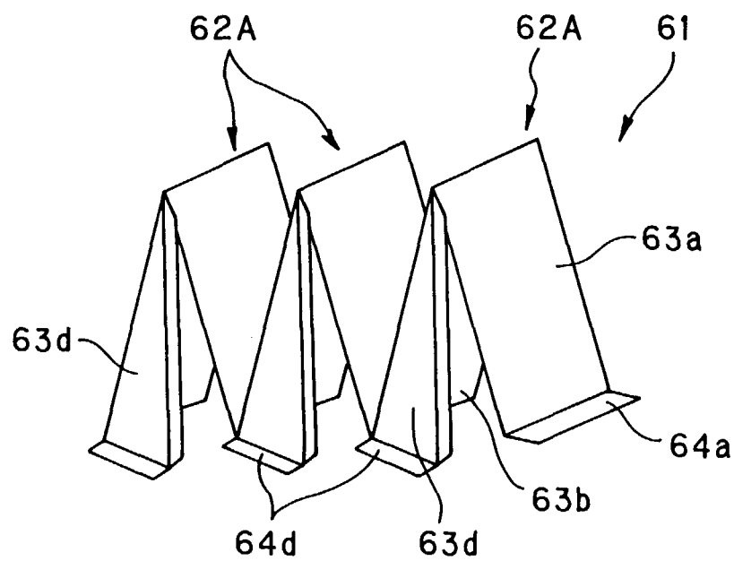
FIG. 28A
