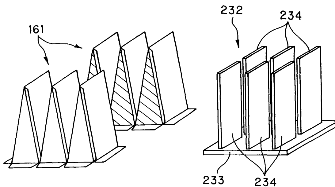
FIG. 29A
