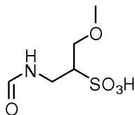
(I-X): 1-formamido-3-methoxypropane-2-sulfonic acid;
