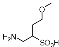
(I-Q): 1-amino-4-methoxybutane-2-sulfonic acid;
