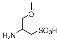
(I-S): 2-amino-3-methoxypropane-1-sulfonic acid;
