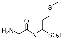
(I-Y): 1-(2-aminoacetamido)-3-(methylthio)propane-1-sulfonic acid;
