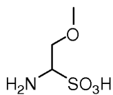
(I-U): 1-amino-2-methoxyethanesulfonic acid;
