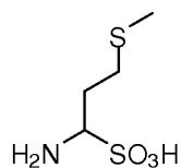
(I-C): 1-amino-3-(methylthio)propane-1-sulfonic acid;
