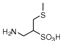
(I-K): 1-amino-3-(methylthio)propane-2-sulfonic acid;
