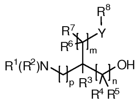
(SI-A)
