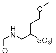
(I-R): 1-formamido-4-methoxybutane-2-sulfonic acid;
