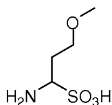
(I-O): 1-amino-3-methoxypropane-1-sulfonic acid;
