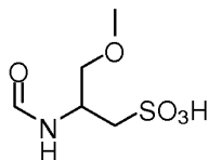
(I-T): 2-formamido-3-methoxypropane-1-sulfonic acid;
