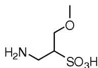
(I-W): 1-amino-3-methoxypropane-2-sulfonic acid;
