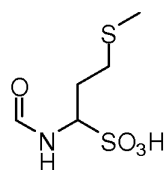
(I-D): 1-formamido-3-(methylthio)propane-1-sulfonic acid;
