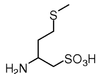
(I-A): 2-amino-4-(methylthio)butane-1-sulfonic acid;
