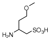
(I-M): 2-amino-4-methoxybutane-1-sulfonic acid;
