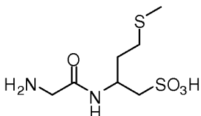
(I-Z): 2-(2-aminoacetamido)-4-(methylthio)butane-1-sulfonic acid;
