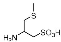
(I-G): 2-amino-3-(methylthio)propane-1-sulfonic acid;
