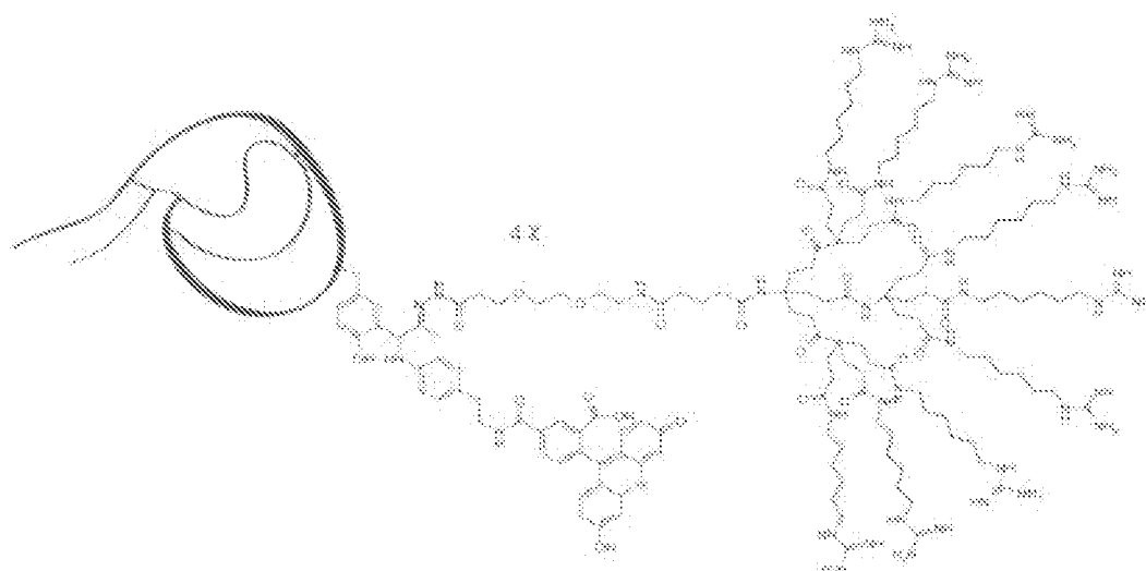
Aprotinin-Fluorophore-Transporter Conjugate
