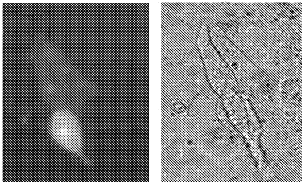
Aprotinin-Fluorophore-Transporter Conjugate
