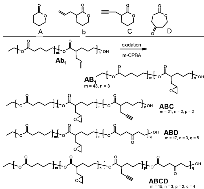
Scheme 5a. Linear precursor.
