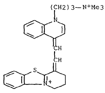
Iodure de Pyrido[2,1-b]benzothiazolium, 1,2,3,4-tétrahydro-4-[[1-[3-(triméthylammonio)propyl]-4(1H)-quinolinylidène]éthylidène]
