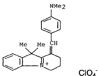
Perchlorate de 6H-Pyrido[1,2-a]indolium, 9-[[4-(diméthylamino)phényl]méthylène]-7,8,9,10-tétrahydro-10,10-diméthyl
