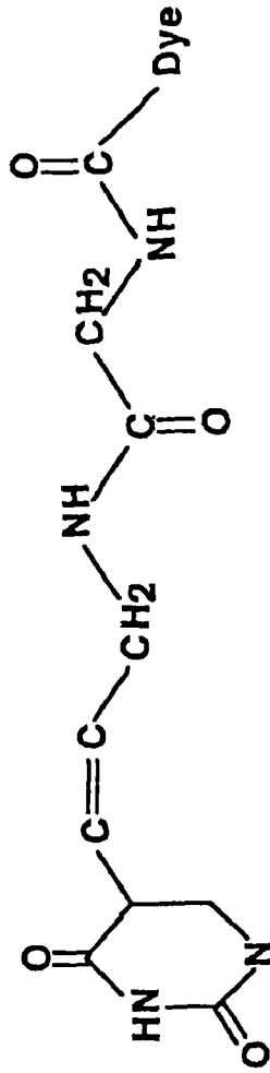
Diglycinyllinker
