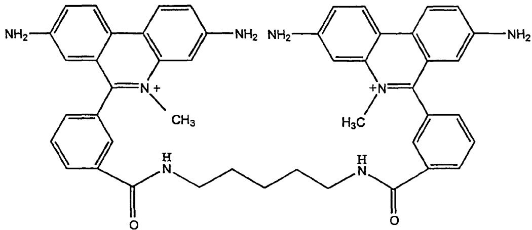
meta -EthD
