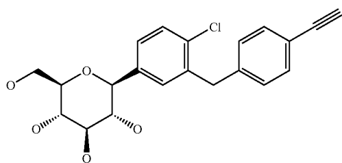
1-Chloro-2-(4-ethynyl-benzyl)-4-(β-D-glucopyranos-1-yl)-benzene
