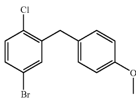
1-Bromo-4-chloro-3-(4-methoxy-benzyl)-benzene
