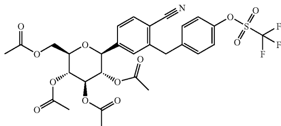
1-Chloro-2-(4-ethyl-benzyl)-4-(β-D-glucopyranos-1-yl)-benzene
