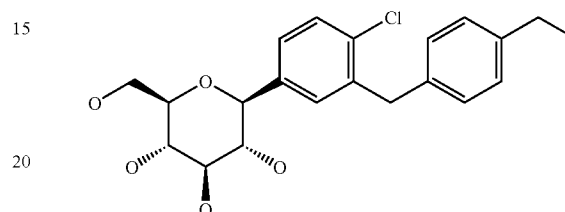
1-Chloro-2-(4-ethyl-benzyl)-4-(β-D-glucopyranos-1-yl)-benzene
