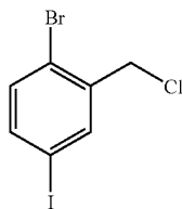
4-Bromo-3-chloromethyl-1-iodo-benzene
