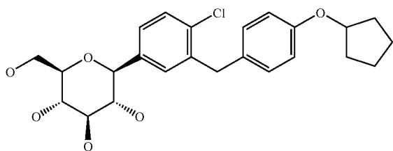
1-Chloro-2-(4-cyclopentyloxybenzyl)-4-(β-D-glucopyranos-1-yl)-benzene
