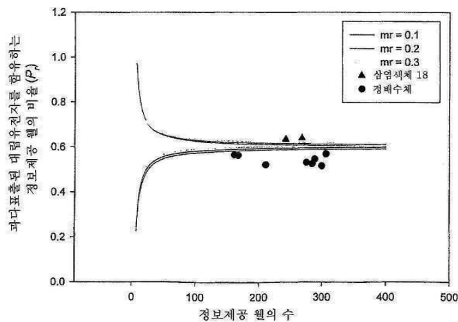
도면16b
