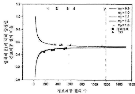
도면14c
