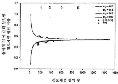
도면14c
