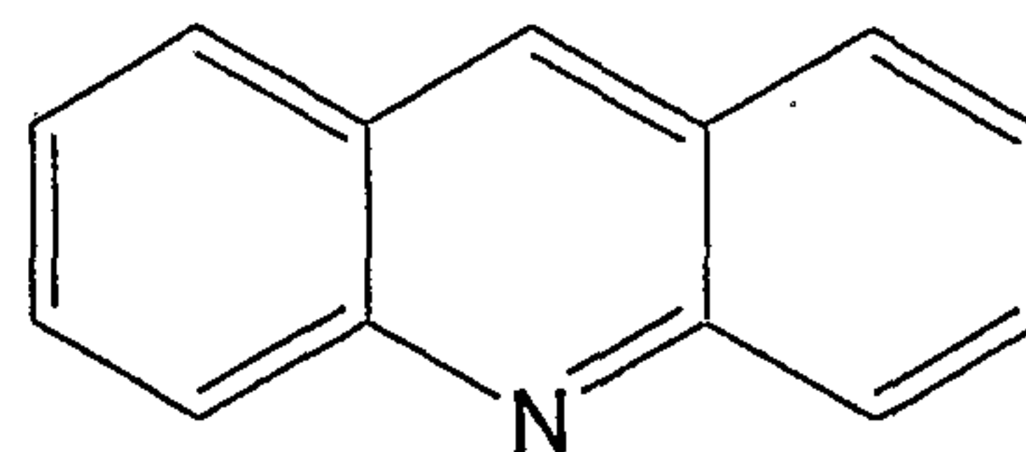
acridine
