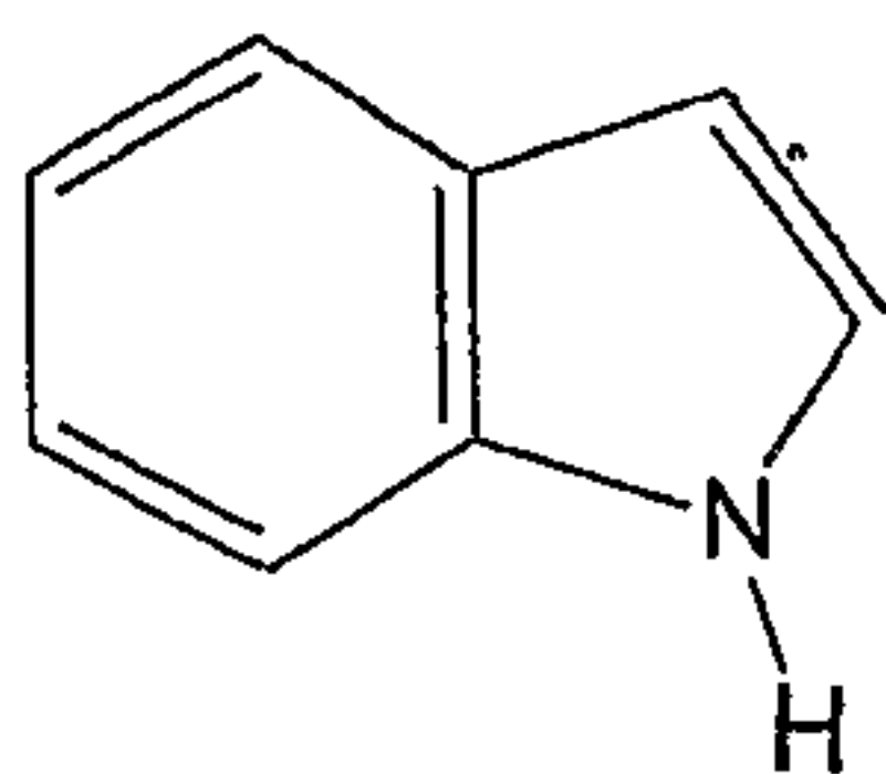
indole
