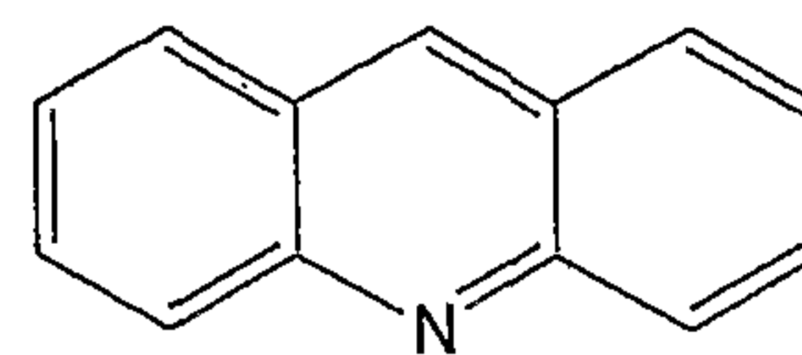
acridine
