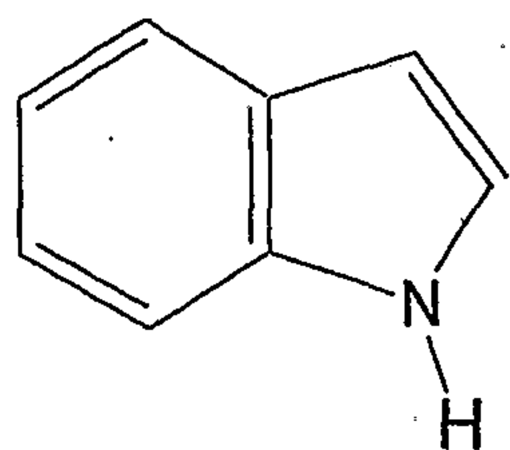
indole
