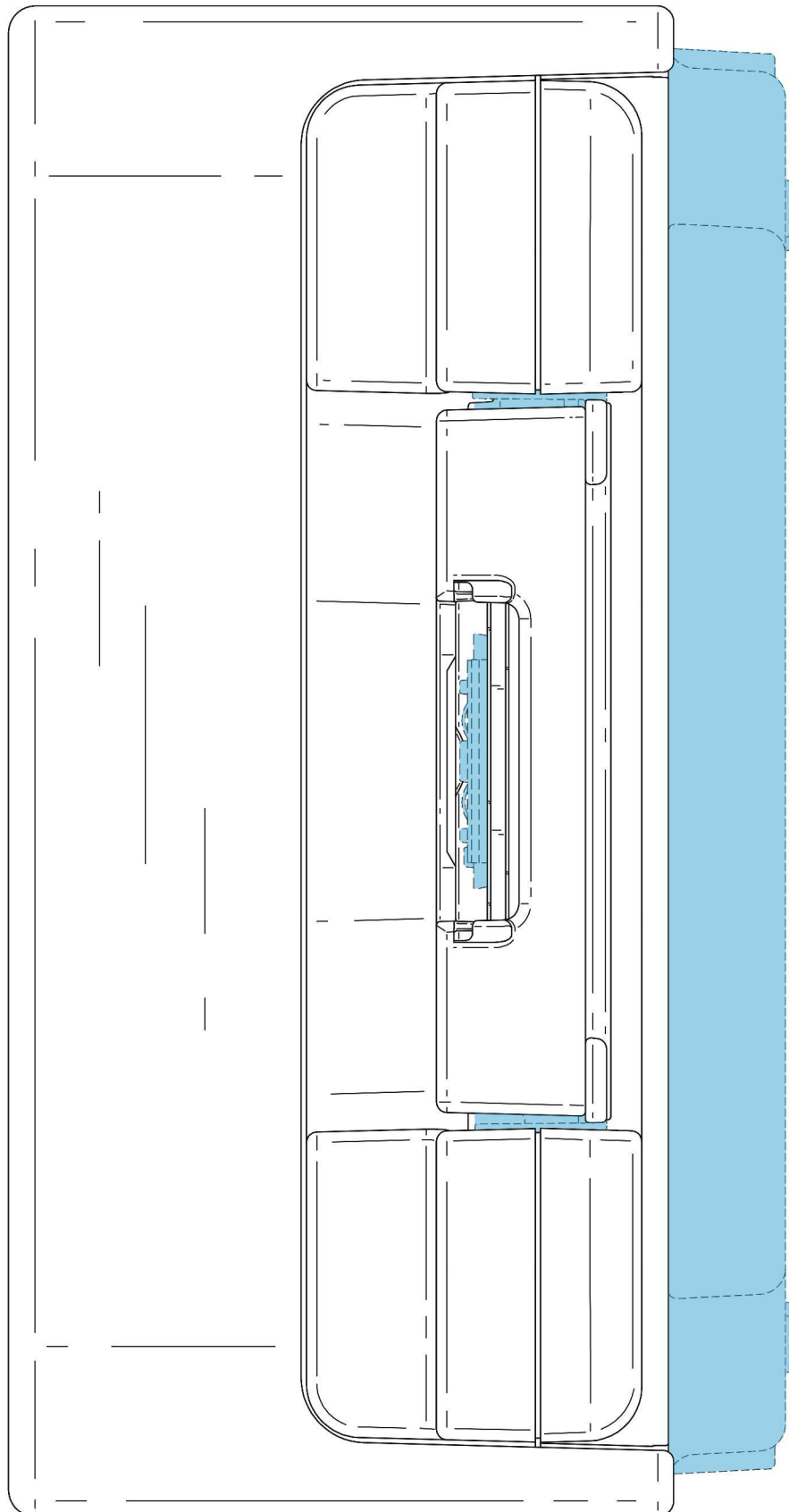
【放大前視圖】
