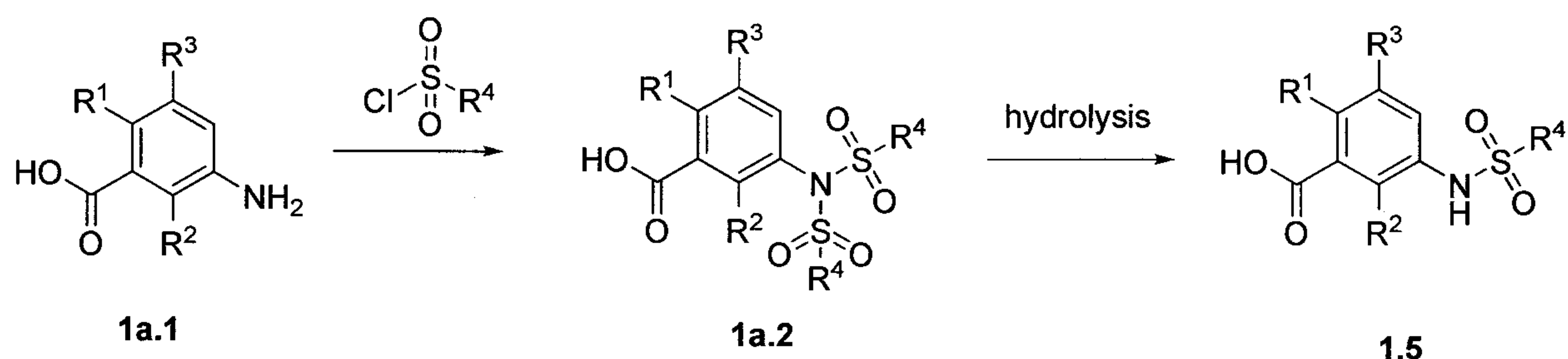
Scheme 1a
