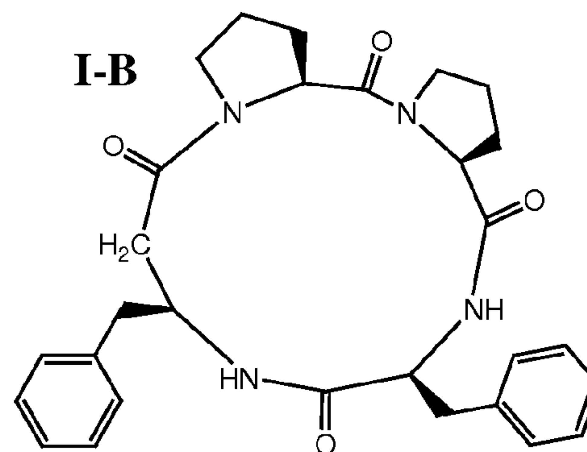
I-B (cyclic(-(L)-Pro-(L)-Pro-(L)-Phe-(L)- \beta^3 hoPhe-)),
