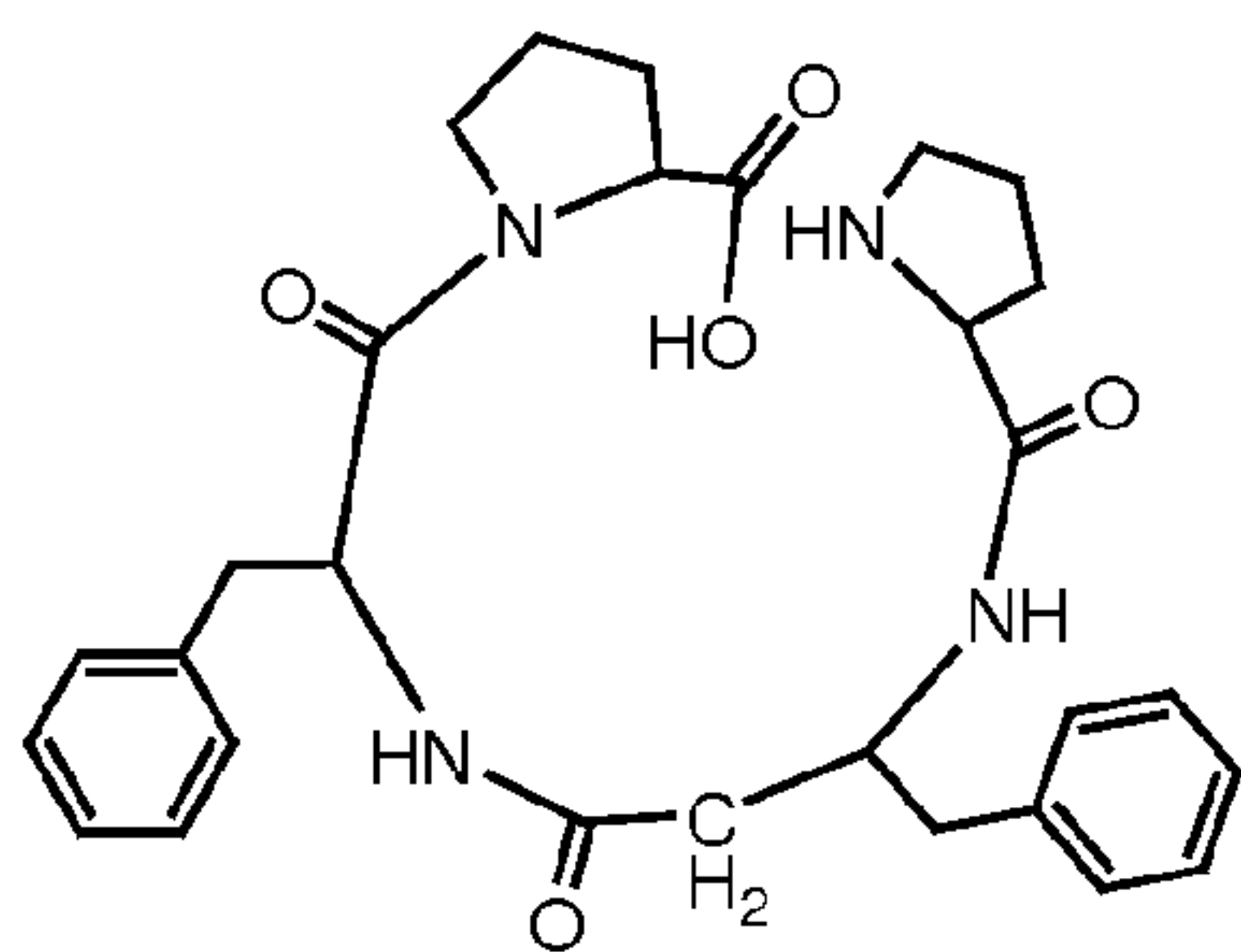
II-4-a (H-Pro-β 3 hoPhe-Phe-Pro-OH),
