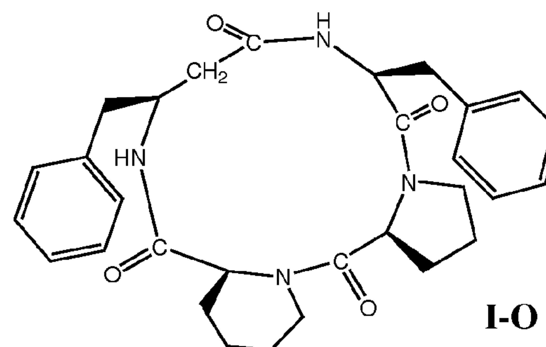
(cyclic(-(L)-Pro-(L)-Pip-(L)- \beta^3 HoPhe-(L)-Phe-)),
