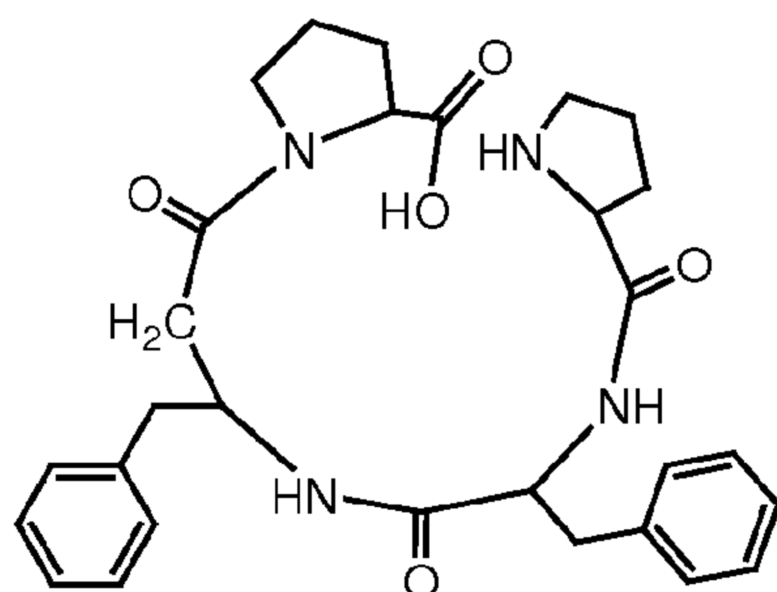
II-4-b (H-Pro-Pro-Phe-β 3 hoPhe-OH),
