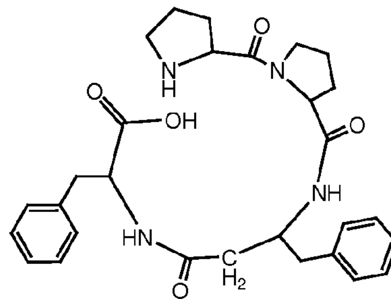
II-1-a (H-Pro-Pro-β 3 hoPhe-Phe-OH),
