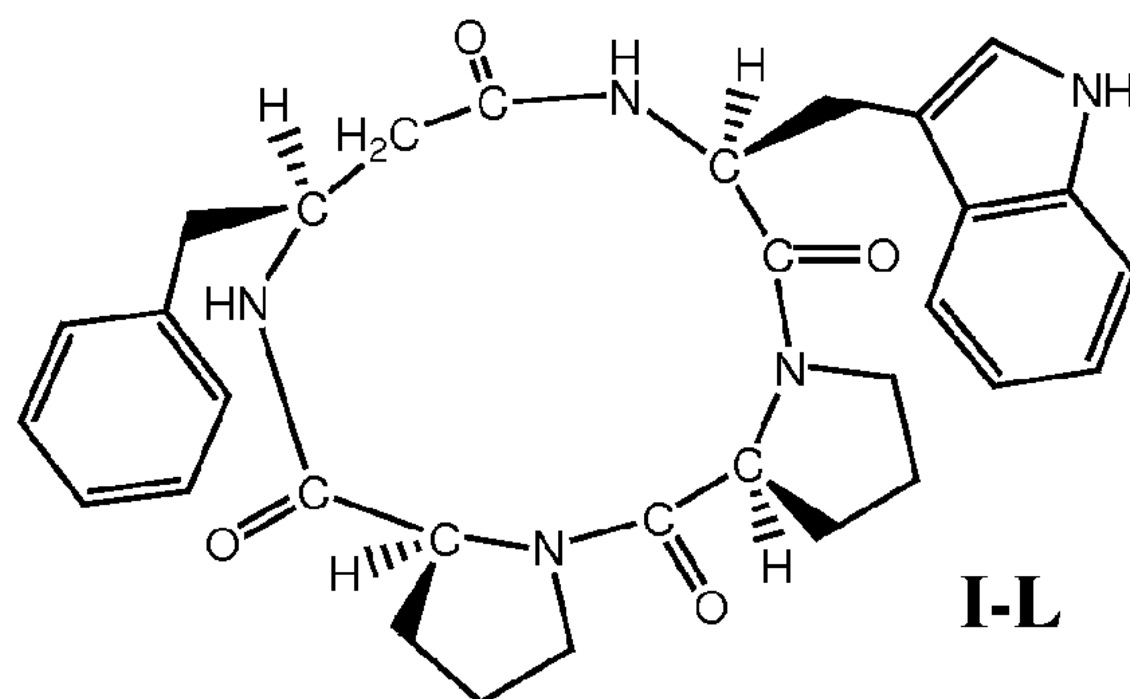
(cyclic(-(L)-Pro-(L)-Pro-(L)- \beta^3 HoPhe-(L)-Trp-)),
