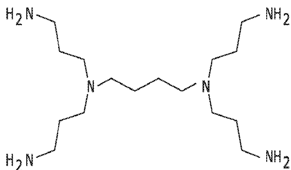
A. G1-NH 2 PPI
