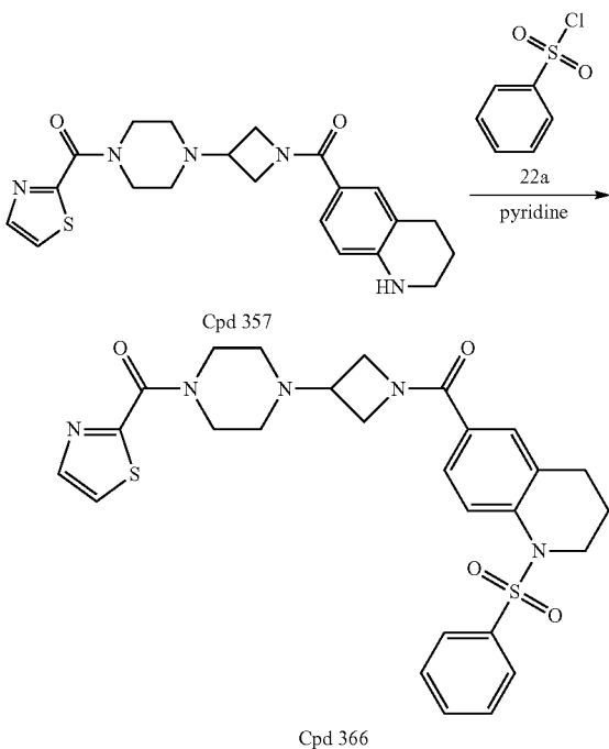
1-(Phenylsulfonyl)-6-({3-[4-(1,3-thiazol-2-ylcarbonyl)piperazin-1-yl]azetidin-1-yl}carbonyl)-1,2,3,4-tetrahydroisoquinoline, Cpd 366
